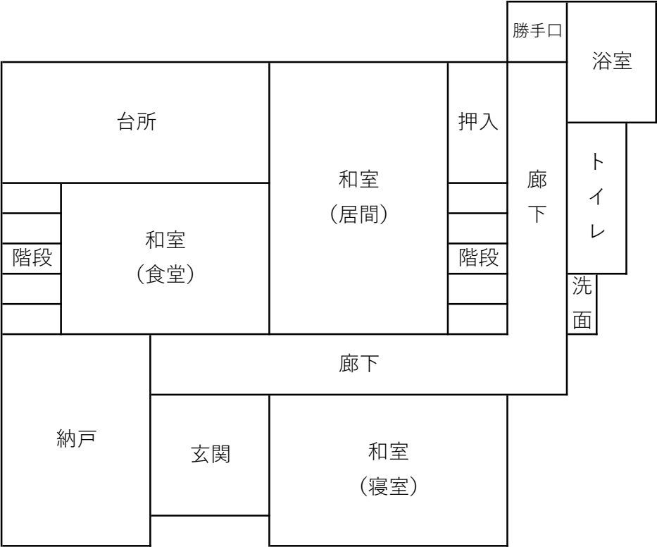
1 階
