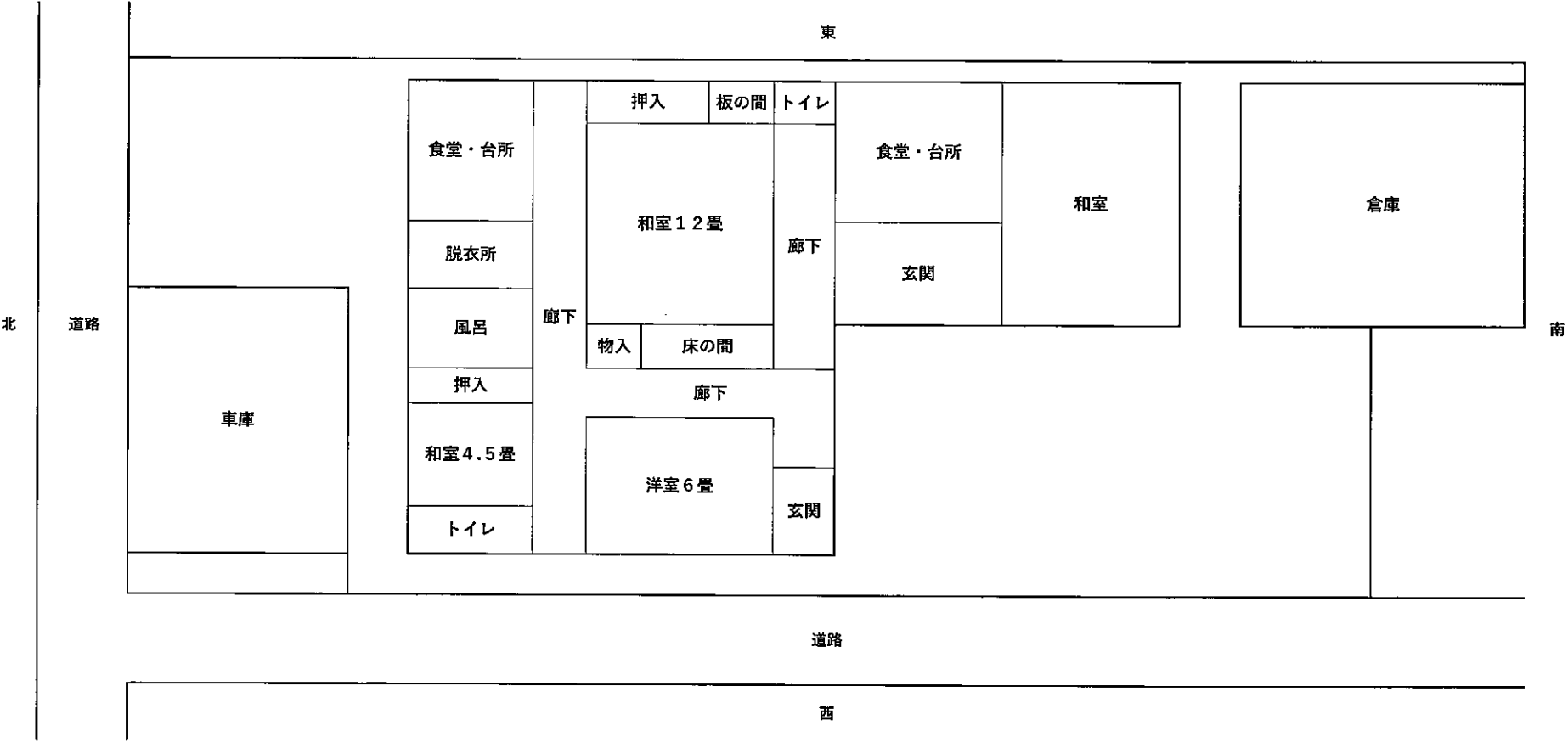
間取り図
